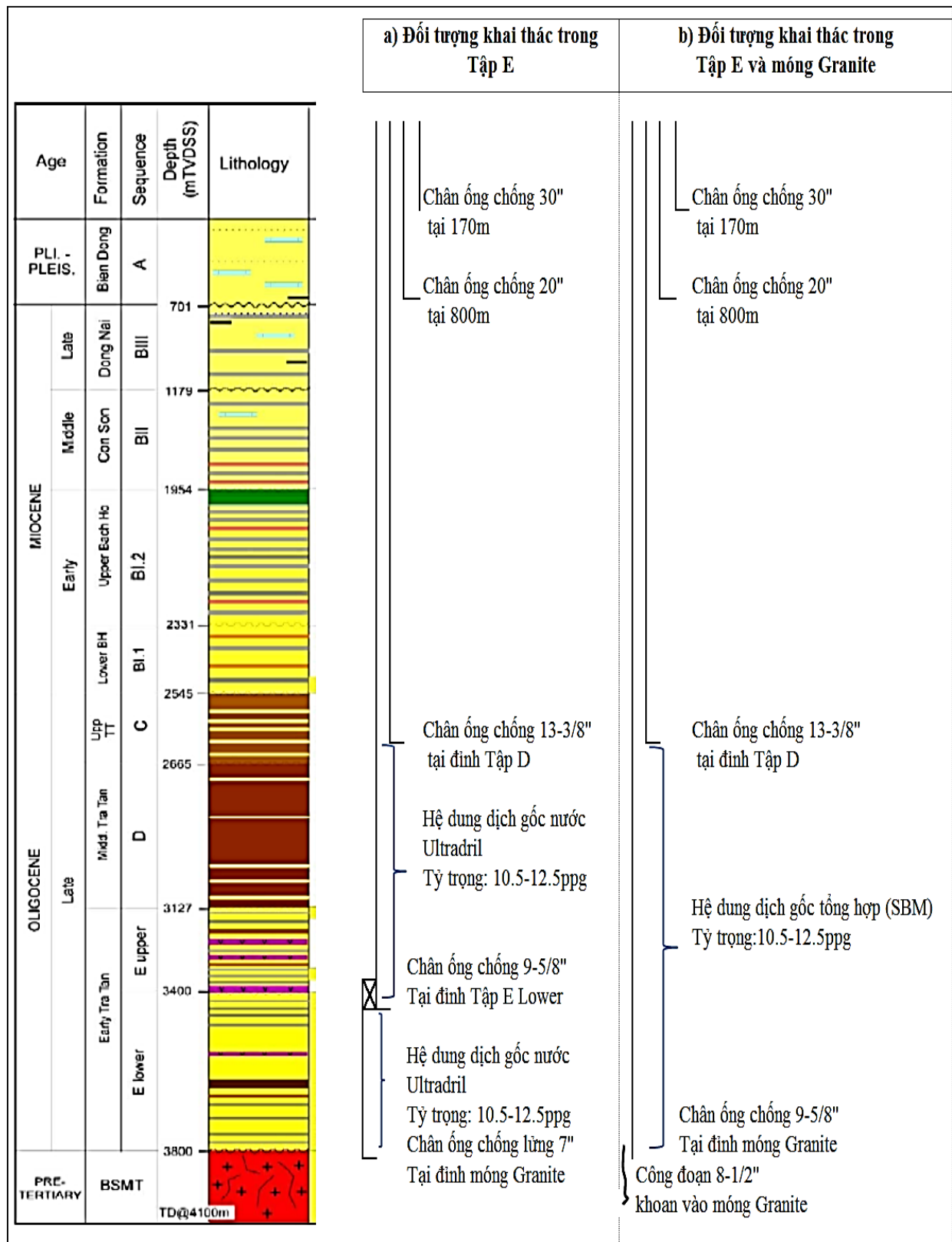
Hình 5. Cấu trúc giếng đề xuất cho các giếng phát triển ở cấu tạo T
