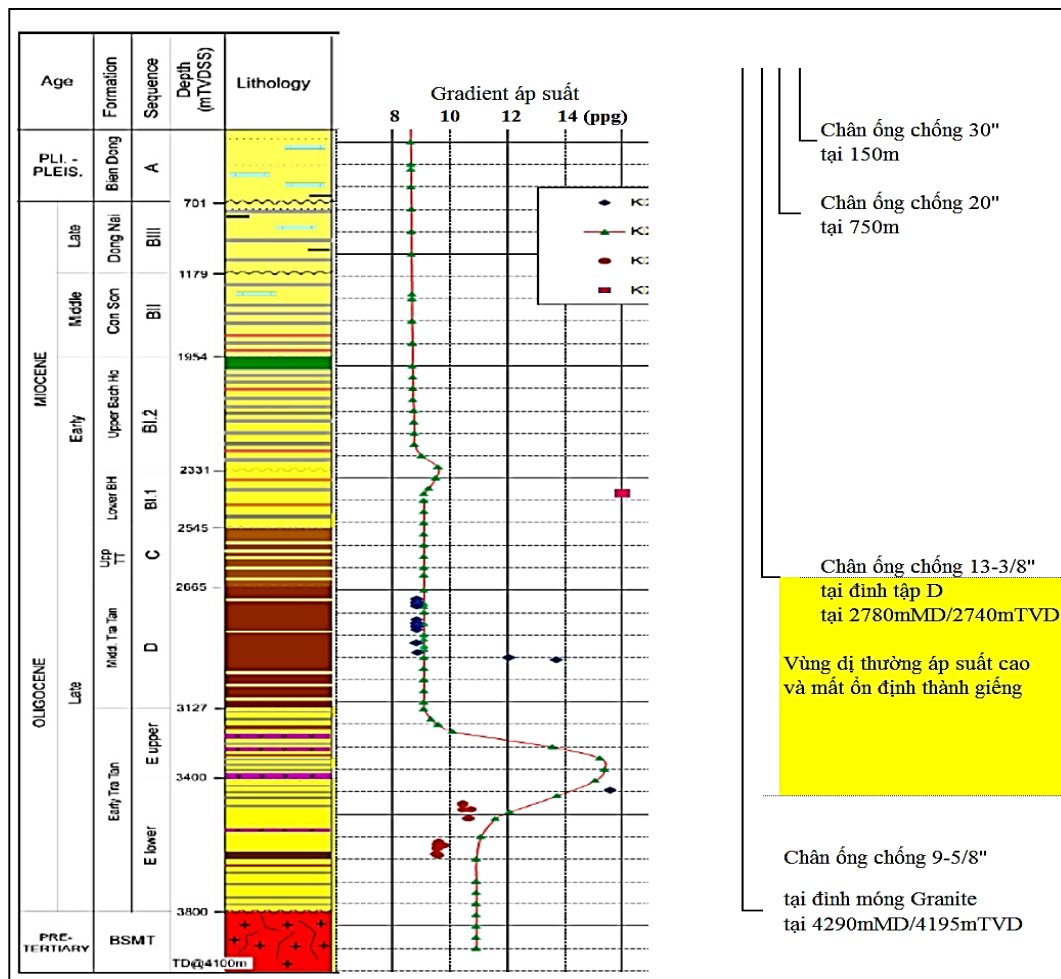
Hình 4. Cấu trúc thiết kế và thực tế sau khi thi công giếng T-3 [4]
