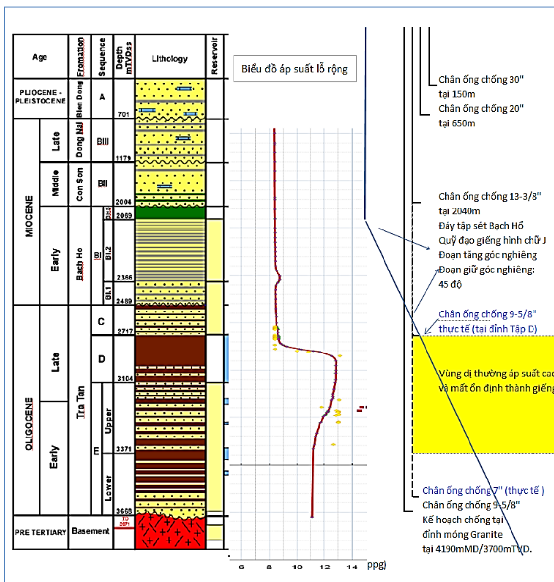
Hình 3. Cấu trúc thiết kế và thực tế sau khi thi công giếng T-2 [4]
