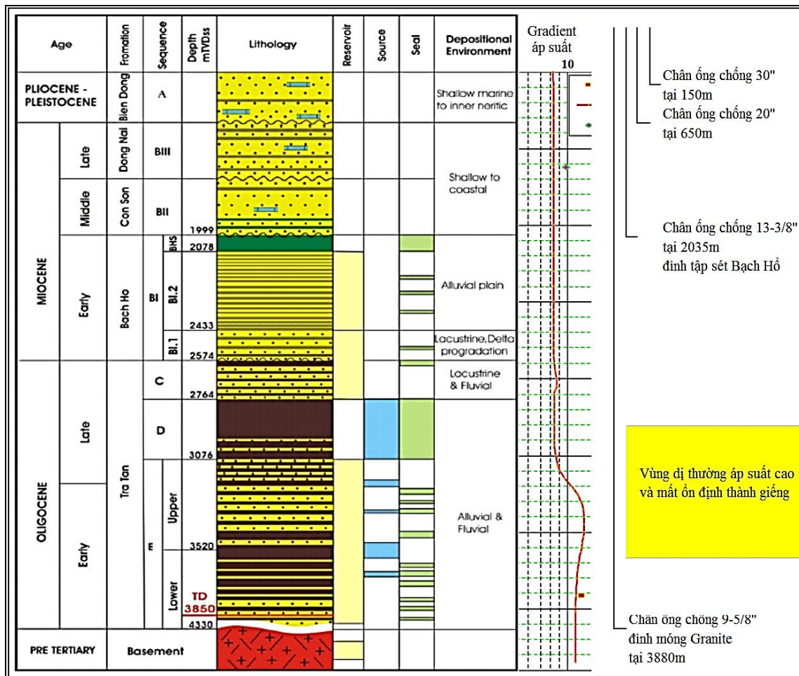
Hình 2. Cấu trúc thiết kế và thực tế sau khi thi công giếng T-1 [4]
