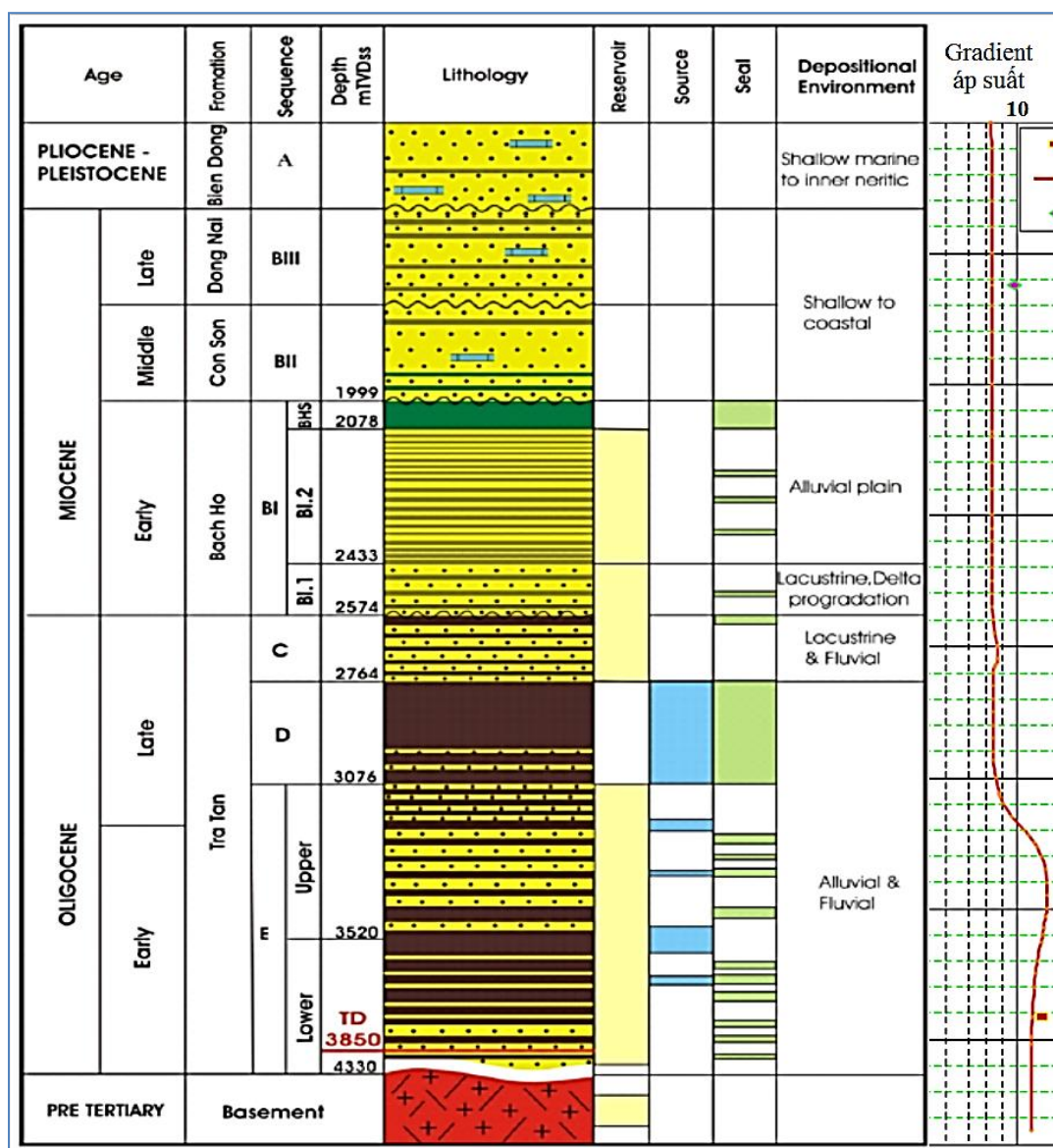
Hình 1. Cột địa tầng tổng hợp của cấu tạo T
